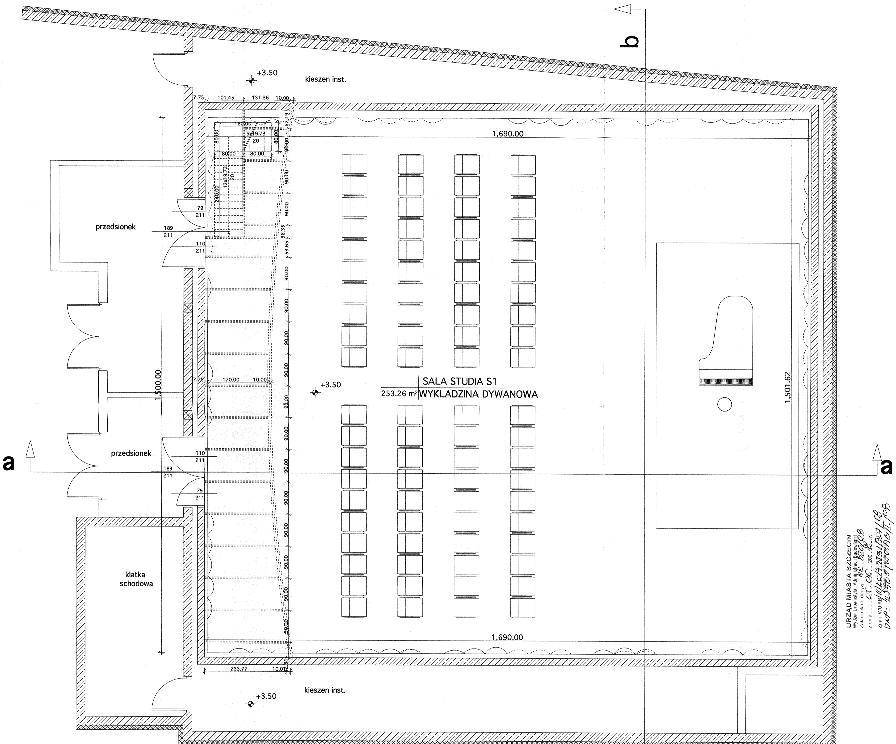
rzut w poziomie podłogi
