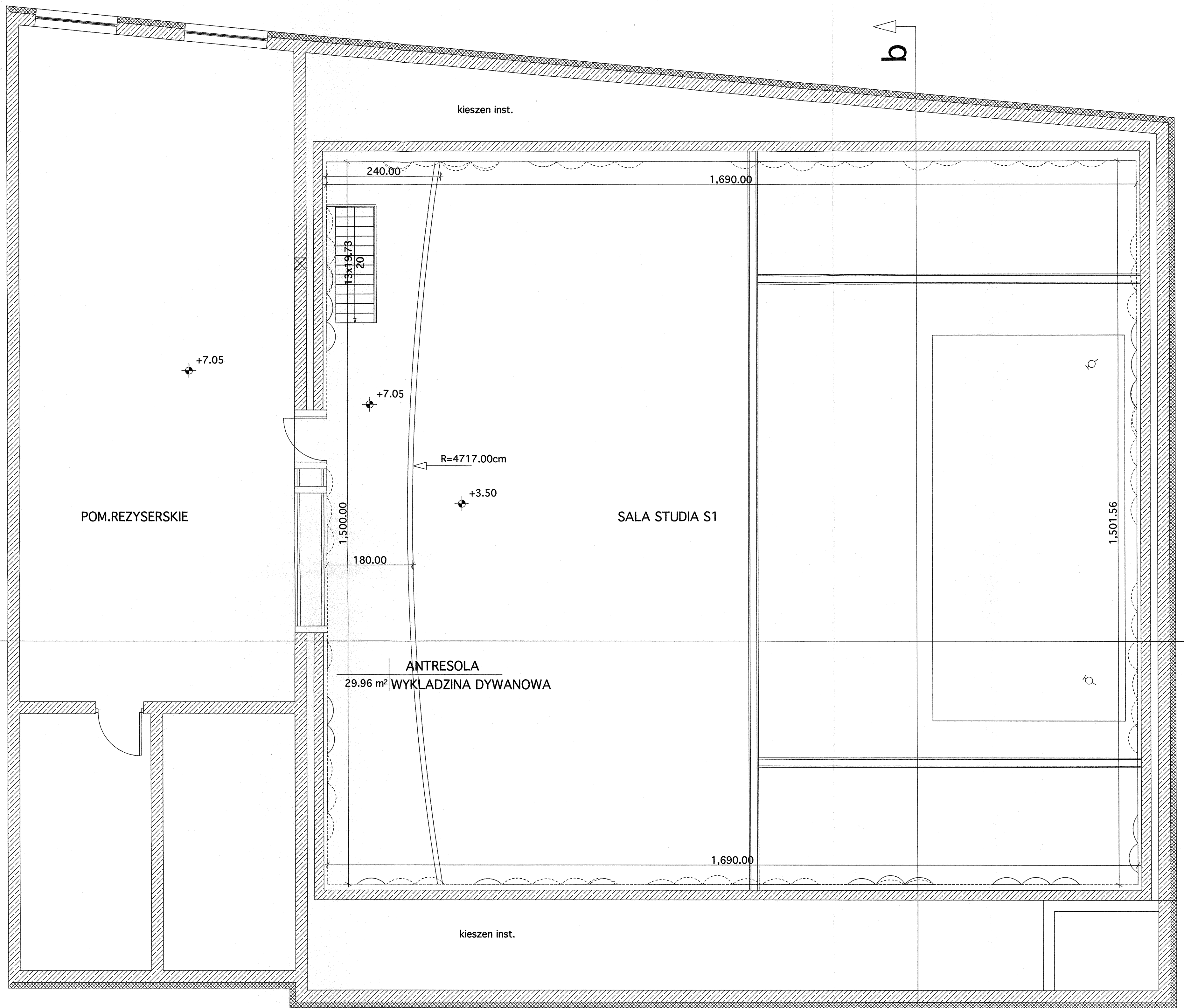
RZUT STUDIA W POZIMIE ANTRESOLI
